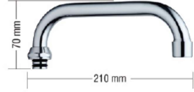
Klasik Döner Eye Borusu 820803
